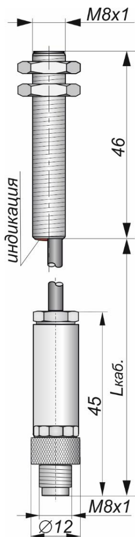
Габаритный чертеж
