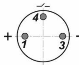
Цоколевка разъема
